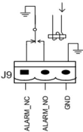
Рис.2-20 Схема разъема сигнала «Ошибка ИБП»
