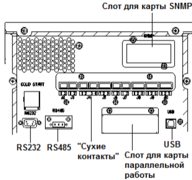
Рис.2-14 Коммуникационные интерфейсы
