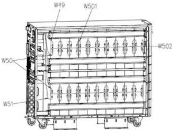
Рис.5-1 Установка батарей
