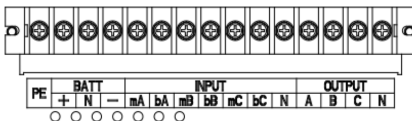
Рис. 2-11 Клеммная колодка на ИБП ЛЕГИОН-3Ф-10-К-Ш/15-20-30-40К-С
